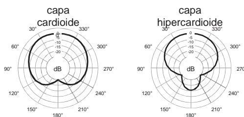
Resposta polar de 1 kHz
